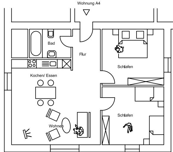
Dachgeschoss
